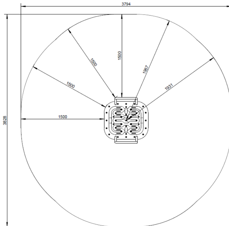
Zeich. Gerät mit Sicherheitszone
