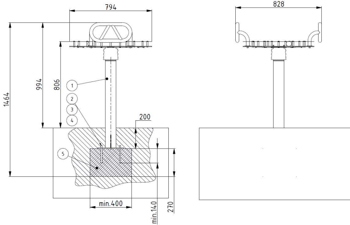
Zeich. Abmessungen des Geräts
